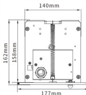
Szczegóły A
